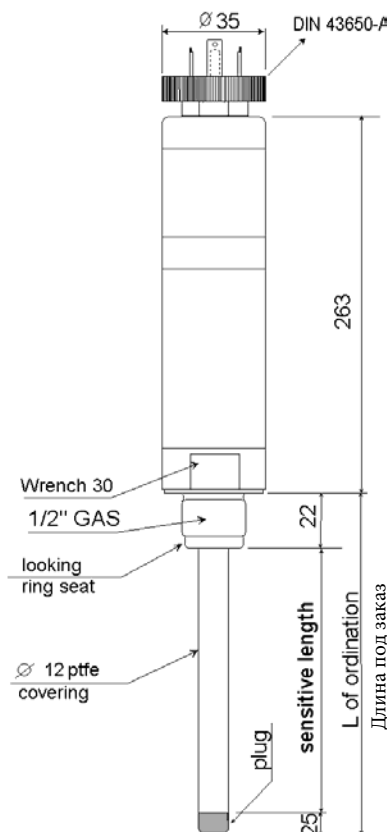
ГАБАРИТНЫЕ РАЗМЕРЫ
